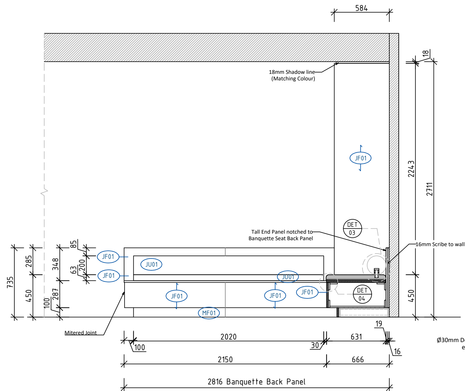
B Elevation Scale: 1:25 @ A3
